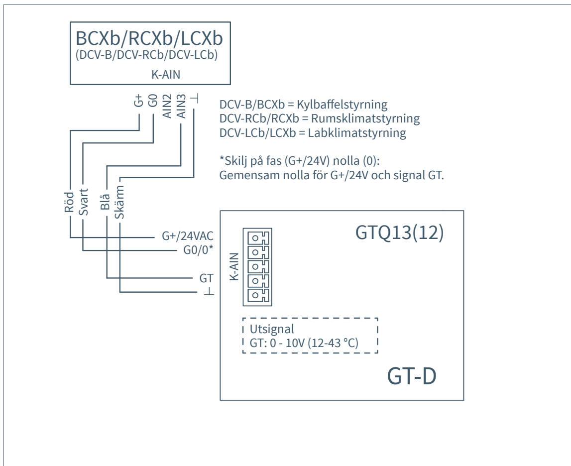
Yttre förbindningsschema GT-D.
