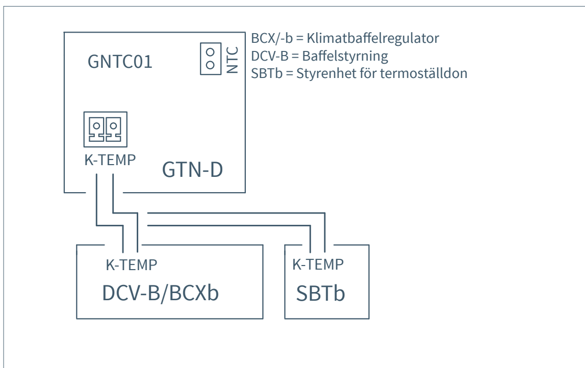
Yttre förbindningsschema GTN-D.
