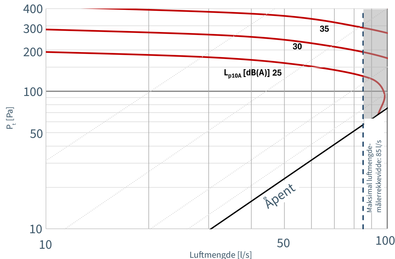
Diagram ICI-F-160, Lydtrykknivå L_{p10A} dB(A)
