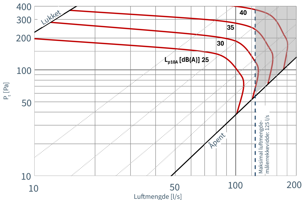
Diagram ICI-F-200, Lydtrykknivå L_{P10A} dB(A)
