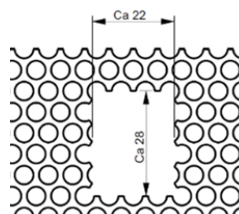
Uttag i raster på kylbaffel.
