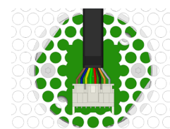
Den monterade sensorenheten. Vy från insida raster ner mot sensor-enhetens baksida.
