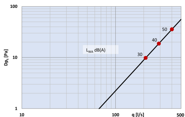
Diagram 5: Total A-vægtet lydeffektniveau, dB(A) for SMID-250
