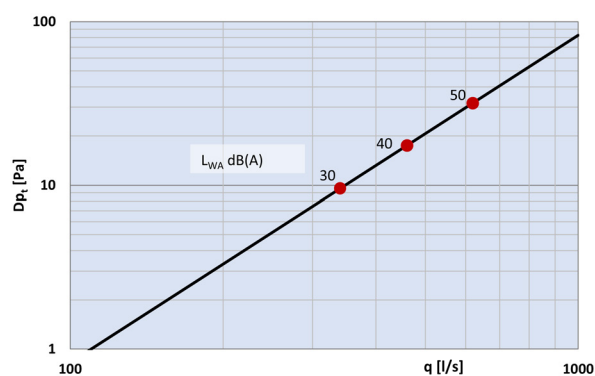
Diagram 6: Total A-vægtet lydeffektniveau, dB(A) for SMID-315
