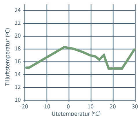
Exempel på tilluftstemperatur för aggregat med roterande värmeväxlare och temperaturoptimering (dimensionerande utetemperatur 25°C).
