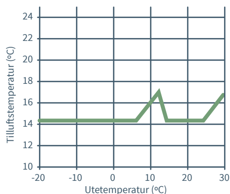
Exempel på tilluftstemperatur för aggregat med vätskekopplade batterier och temperaturoptimering (dimensionerande utetemperatur 25°C).
