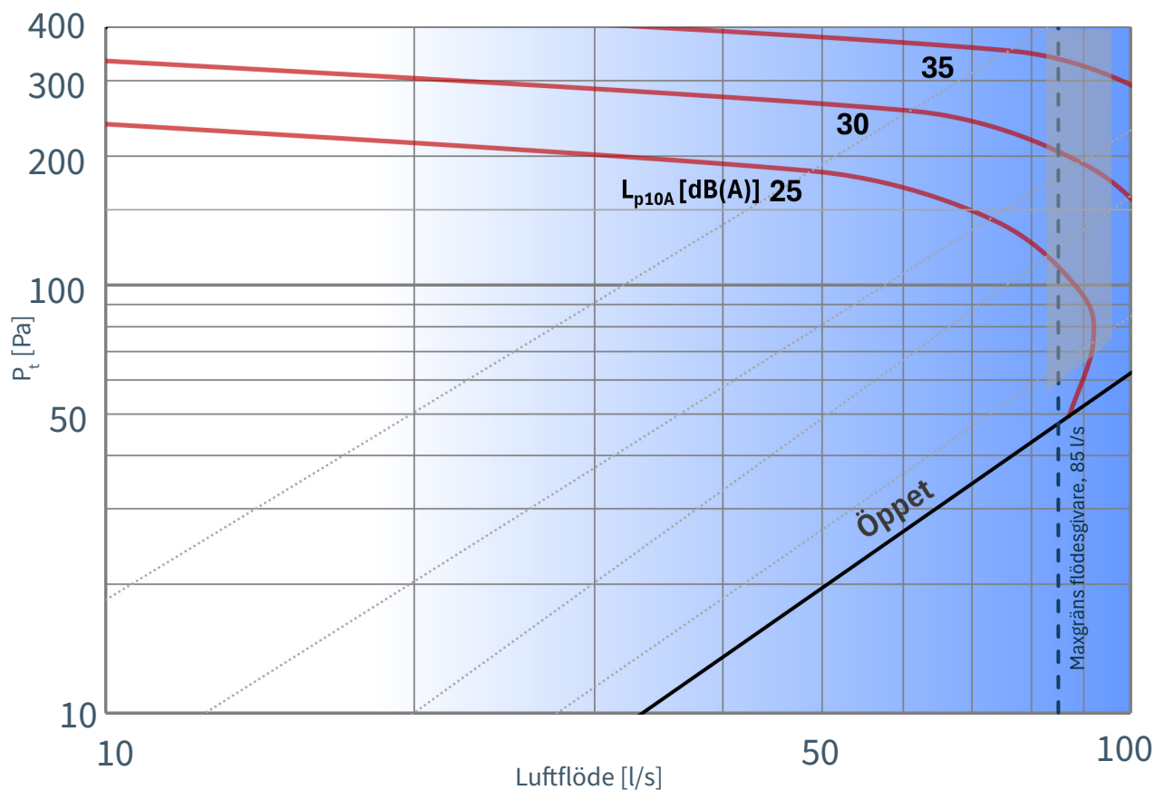
Diagram ISQ-160 från version C, Ljudtrycksnivå L_{P10A} dB(A)
