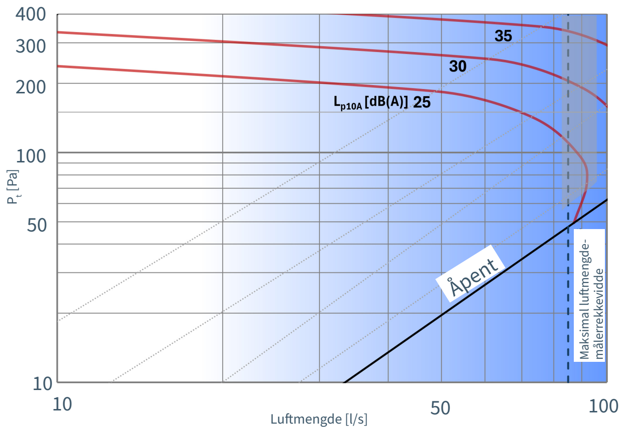
Diagram ISQ-160 version C01, Lydtrykknivå L_{P10A} dB(A)
