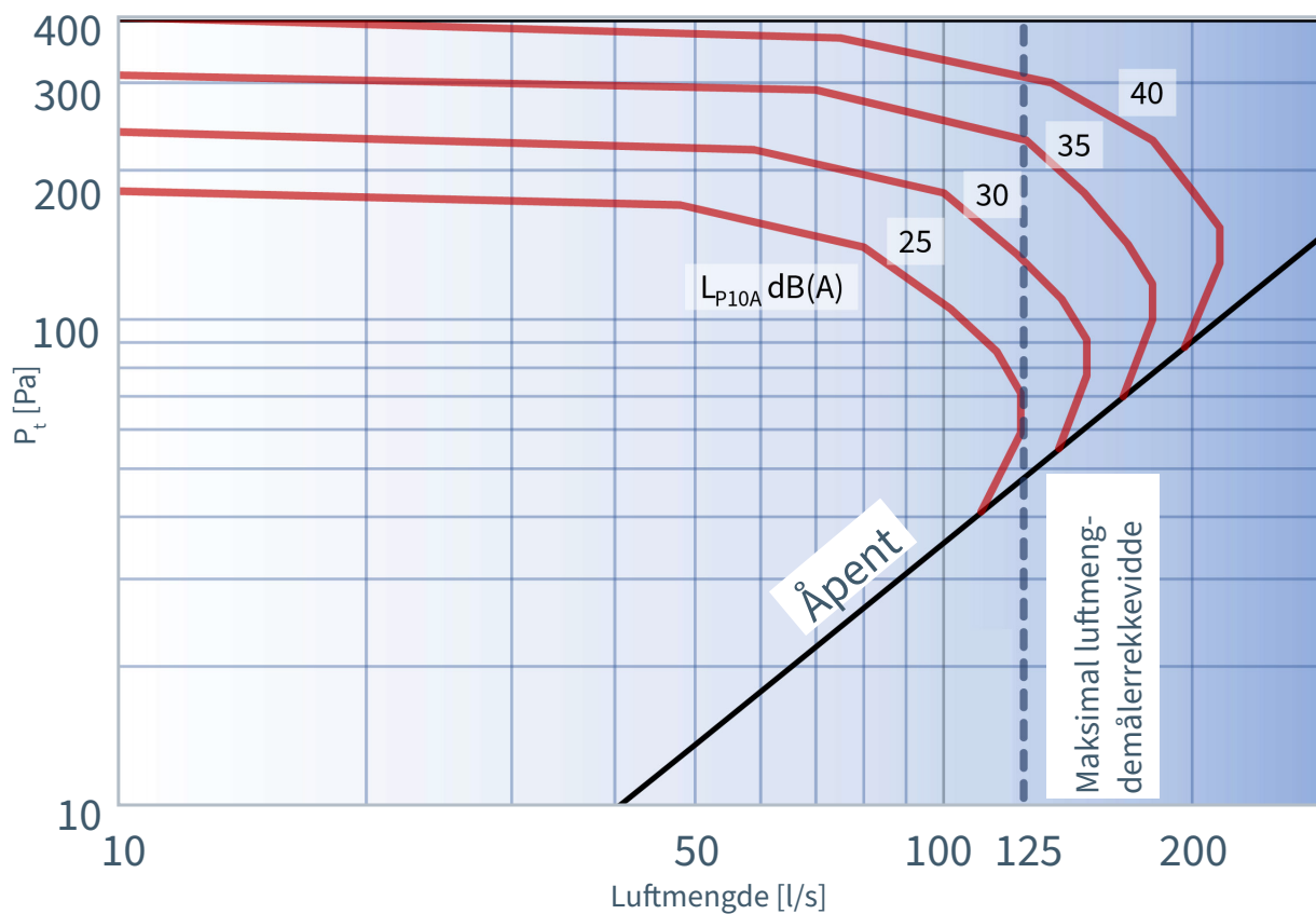
Diagram ISQ-200 fra versjon A01, Lydtrykknivå L_{P10A} dB(A)
