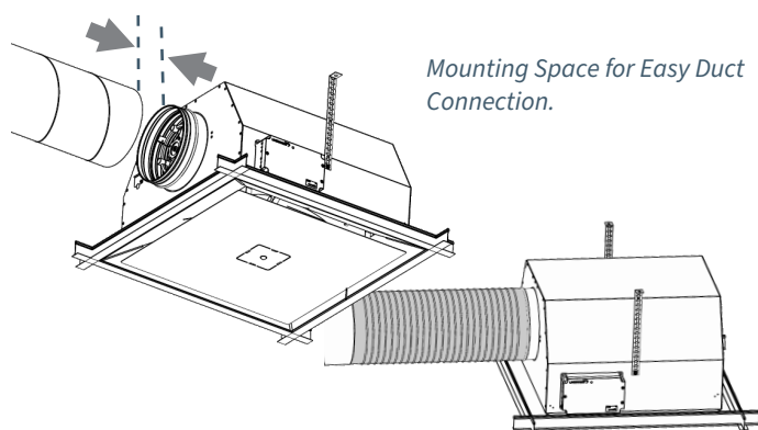
Tilslutning via aluminiumsslange type Drasut.
