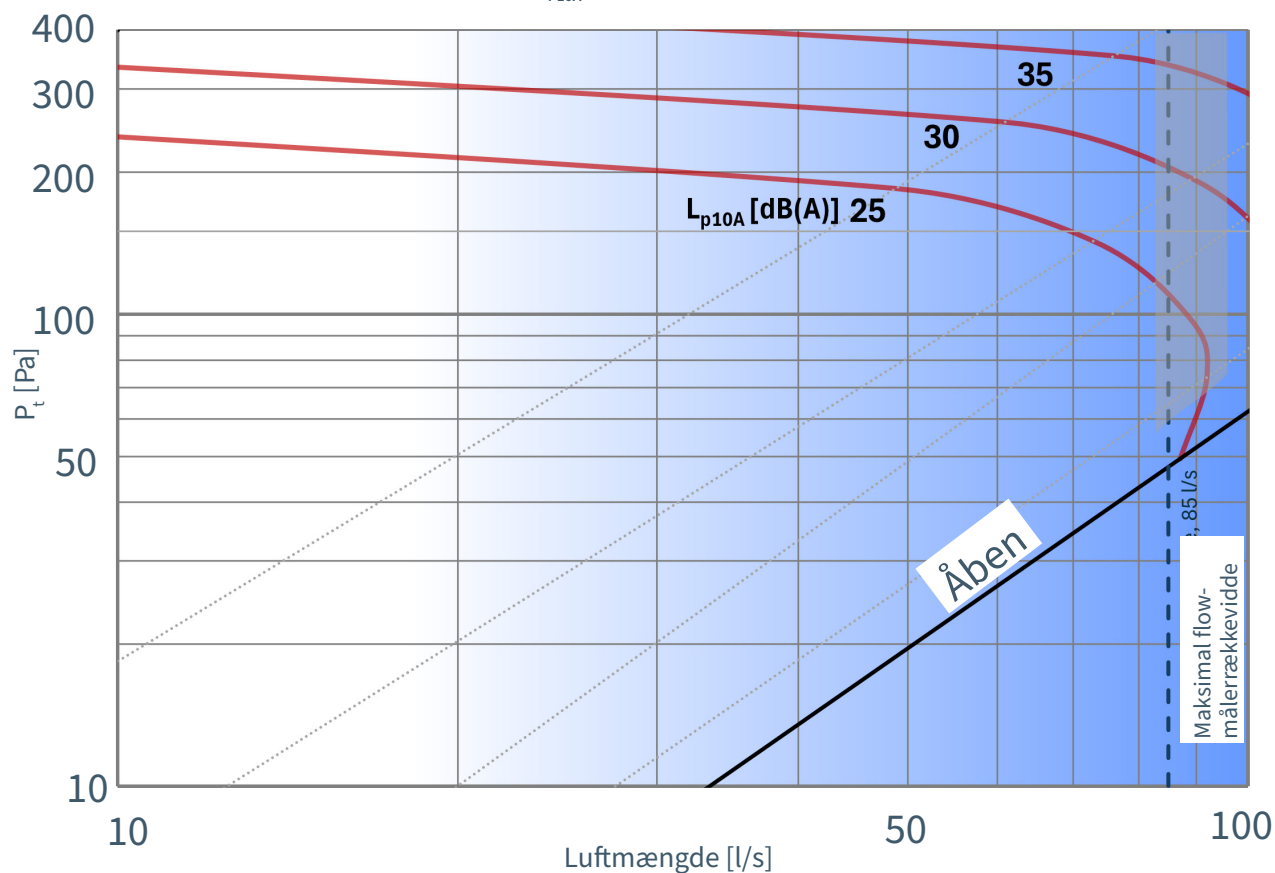
Diagram ISQ-160 fra version C, Lydtryksniveau L_{P10A} dB(A)
