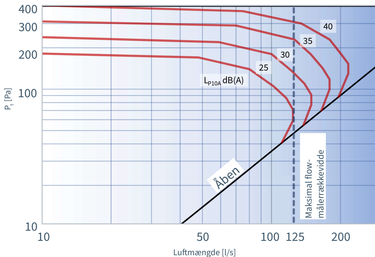
Diagram ISQ-200 fra version A01, Lydtryksniveau L_{P10A} dB(A)
