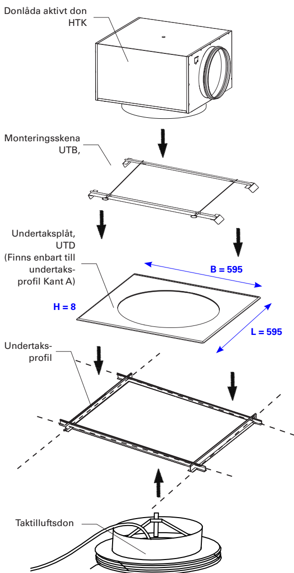
Montage av aktivt taktilluftsdon med undertaksplåt UTD och monteringskena UTB. Mått i mm.
