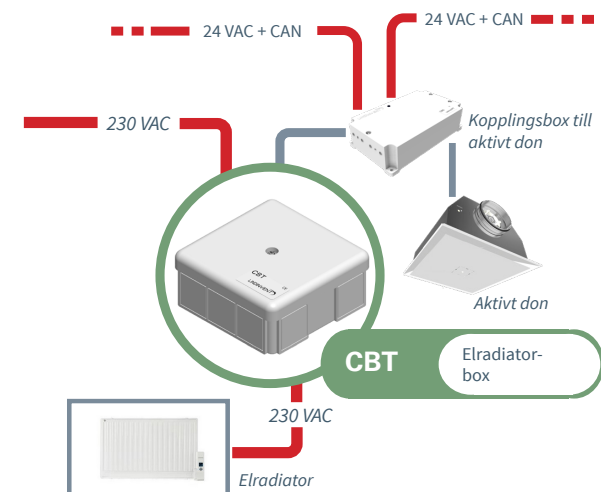
Anslutningsschema CBT.
