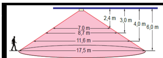
Räckvidd:Maximal vid olika höjder
