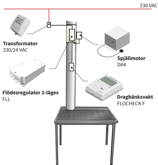
Dragbenk med Flocheck F og øvrige komponenter for strømsstyring.
