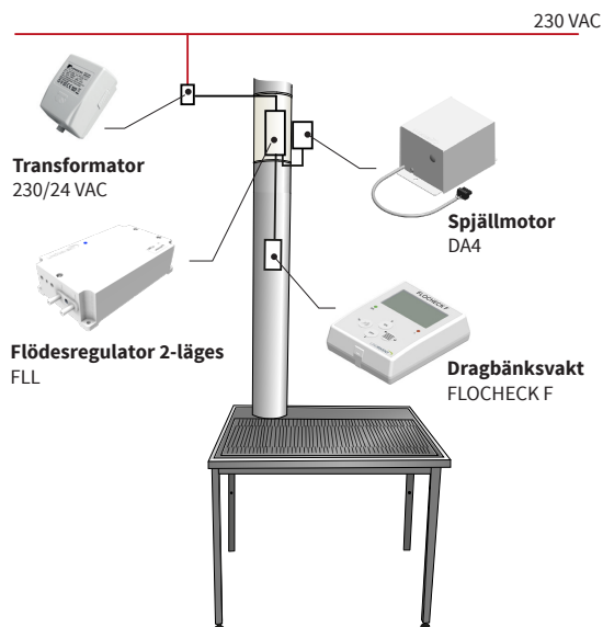
Trækbænk med Flocheck F og øvrige komponenter til strømningsstyring.
