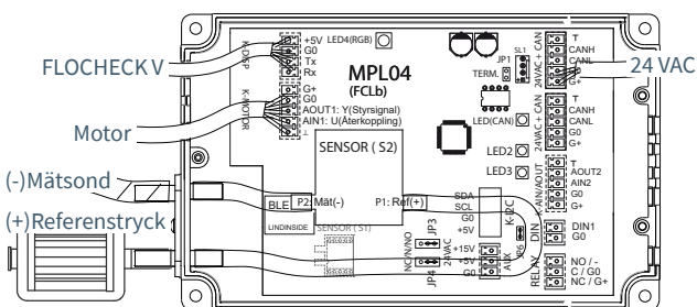
Illustration 11. Inkopplingar på FCLb med markerad kopplingsplint för elförreglingskontaktorn EFK.
