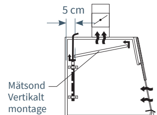
Illustration 3M. Dragskåp med luft-spalt för drag enbart upptill i skåpet: Här placeras mätsonden vertikalt med mät håll riktade rakt in i skåpet mot baksidan.
