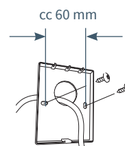
Illustration M3. Montage direkt på vägg/motsvarande.
