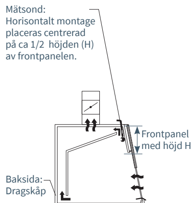
Illustration 2M. Dragskåp med spalt både nedtill och upptill för drag: Mätsonden placeras horisontellt med mät håll riktade rakt in i skåpet mot baksidan.
