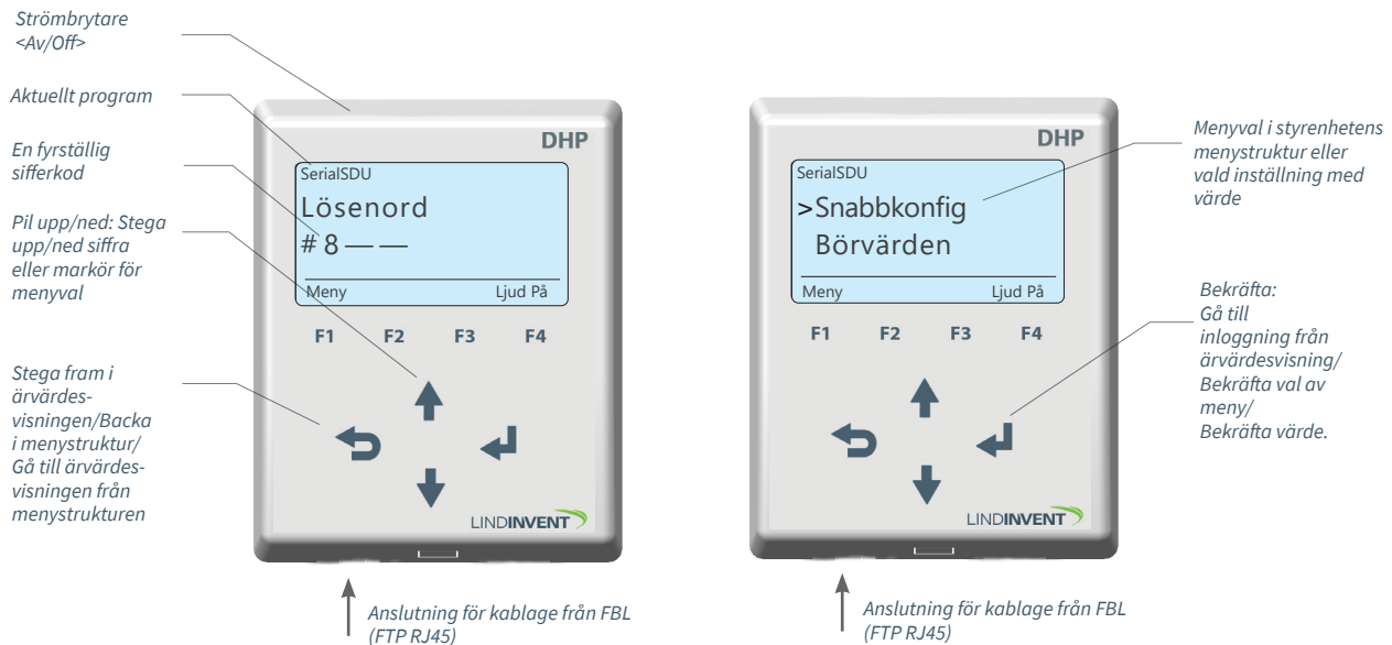
Skärmbilder med förutsättningar före och efter inloggning på en styrenhet via SerialSDU och DHP Version A02.
