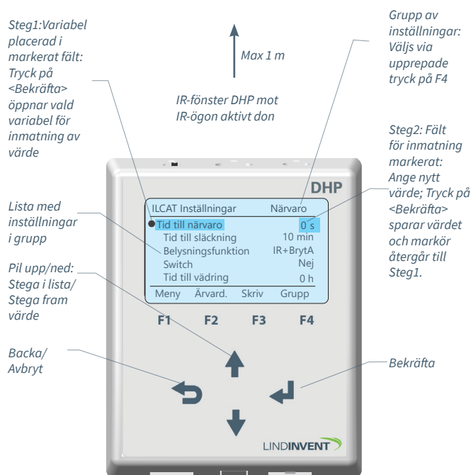
Skärmvy i DHP; ILCAT Inställningar: Funktionsval F3 (Steg3) skriver inmatade värden till tilluftsdonet.
