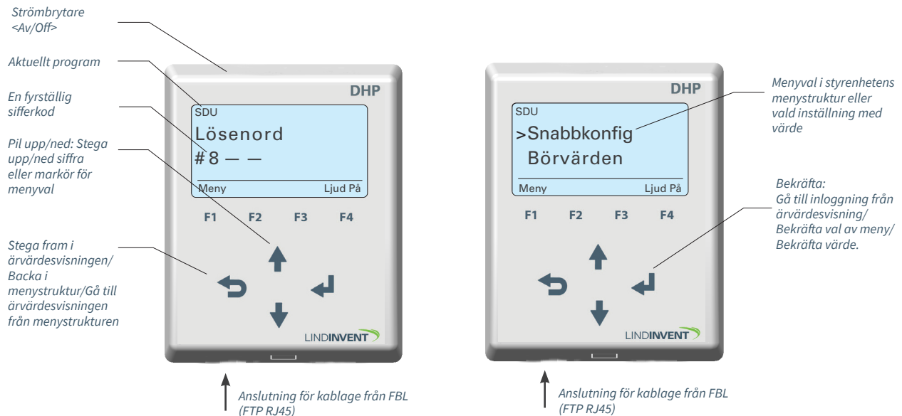
Skärmbilder med förutsättningar före och efter inloggning på en styrenhet via SDU och DHP Version A02.
