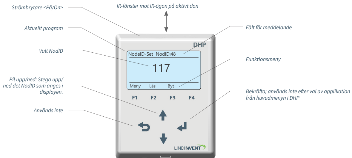
Skärmbild och knappsats i applikationen ILCAT NodeID-Set.
